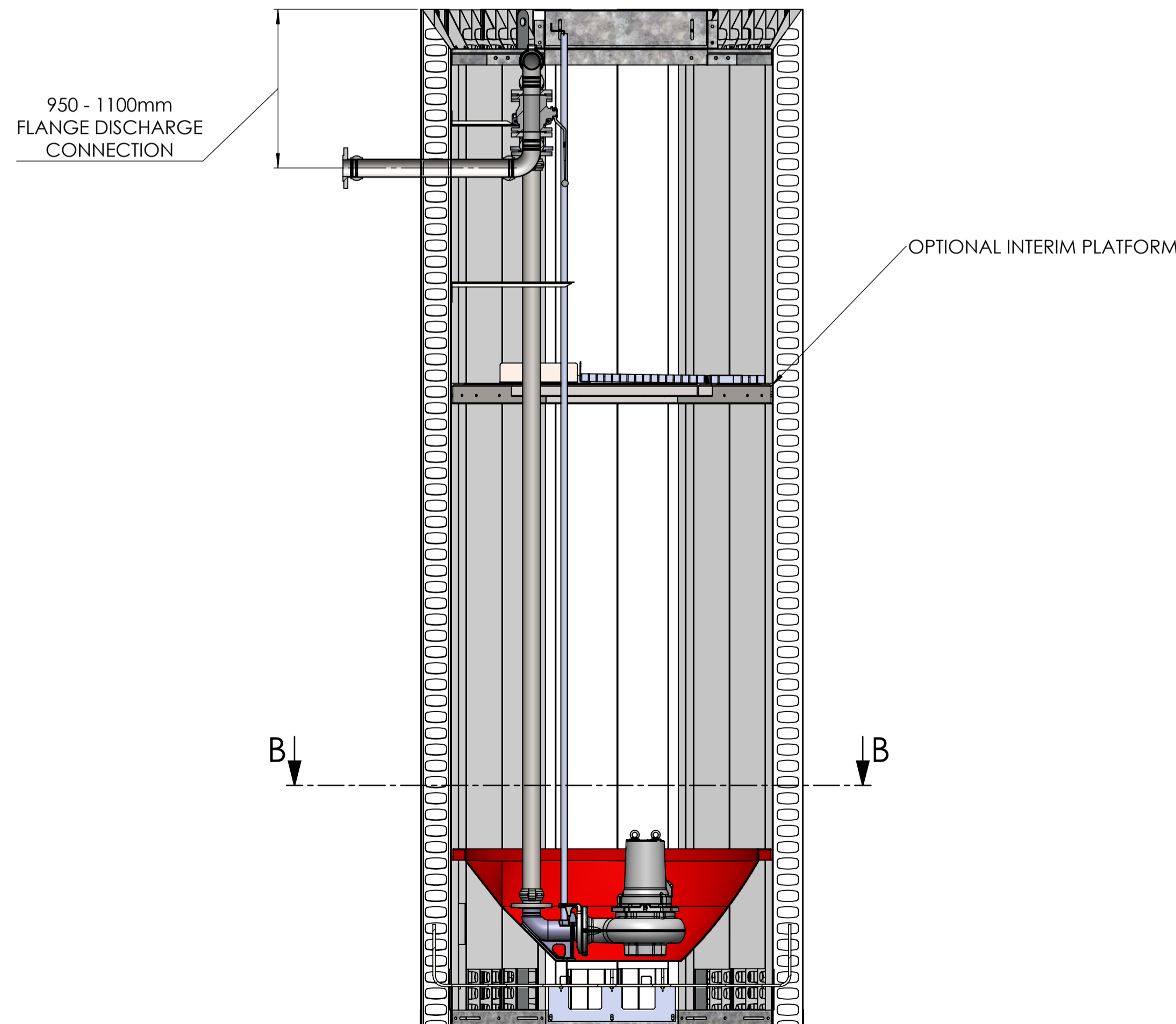
SECTION A-A
